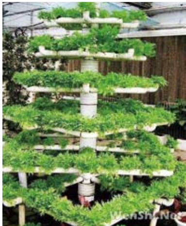
无土栽培营养液管道多层栽培
